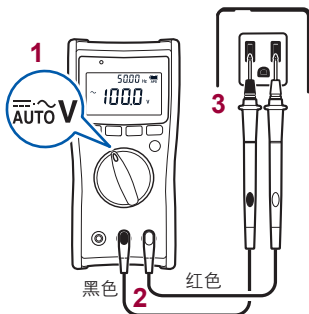
交流电压
