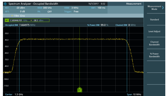
R&S®FPC-K55：占用带宽测量
